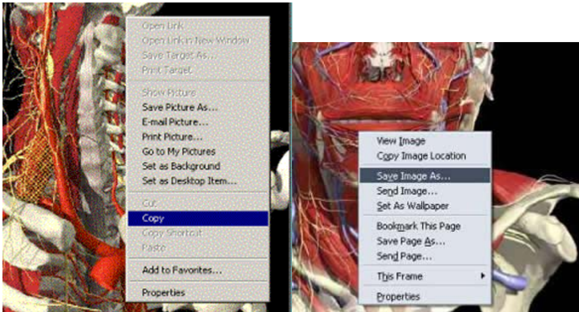
図 1 (Internet Explorer)
