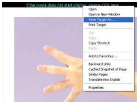
図 3 (Internet Explorer)
